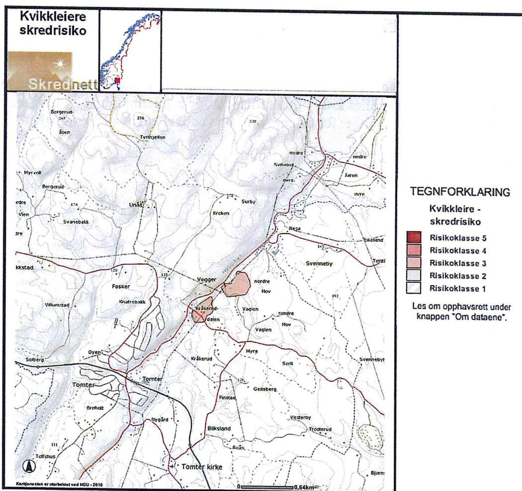
Figur 4: Kartet viser de to eneste områdene hvor det er registrert fare for større leirskred.
