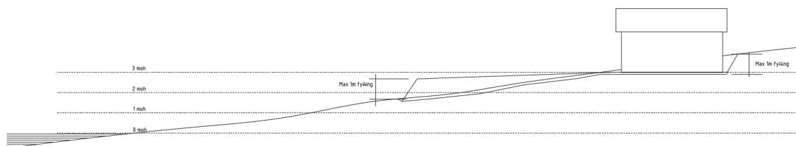
Figur 2 Illustrasjon Snitt Naustområdet. Tillatt fylling/ skjæring
