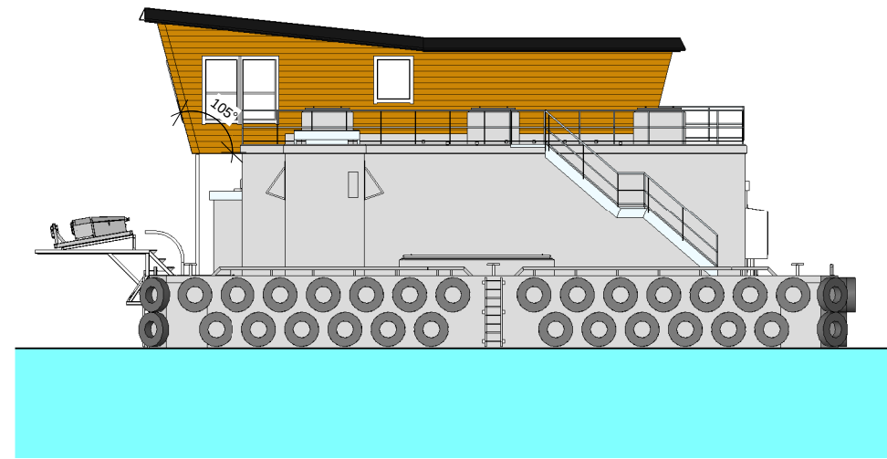
3 FASADE VELFERDSIDE 1 : 200
