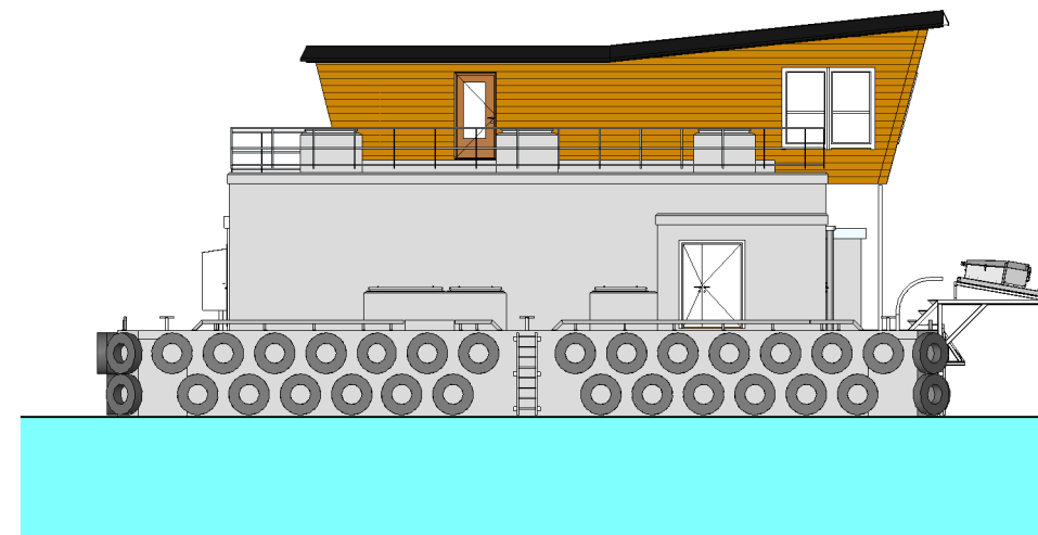
4 FASADE SILOER 1 : 200
